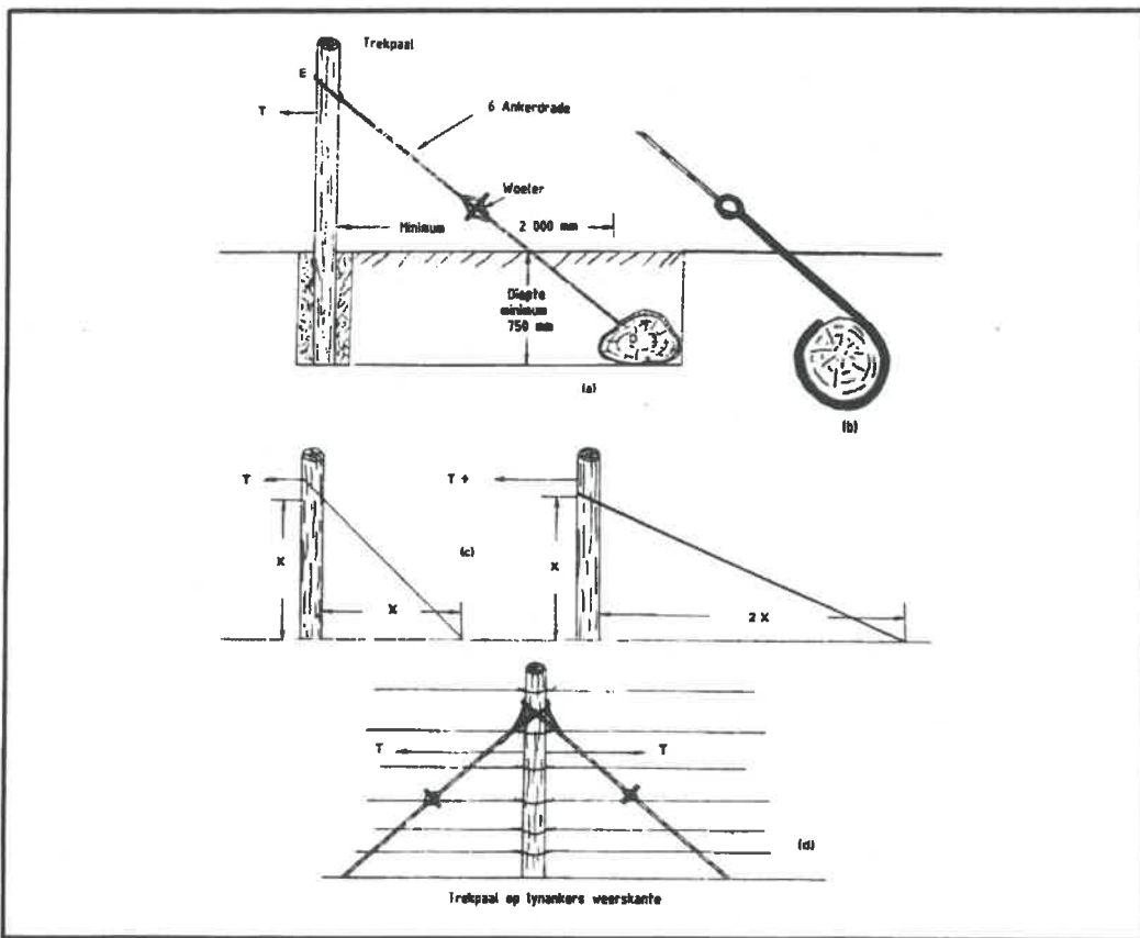
Fig. 5.3: Enkelpaaldraadankers
